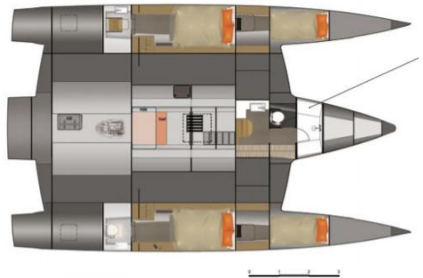
Coque centrale et flotteurs
